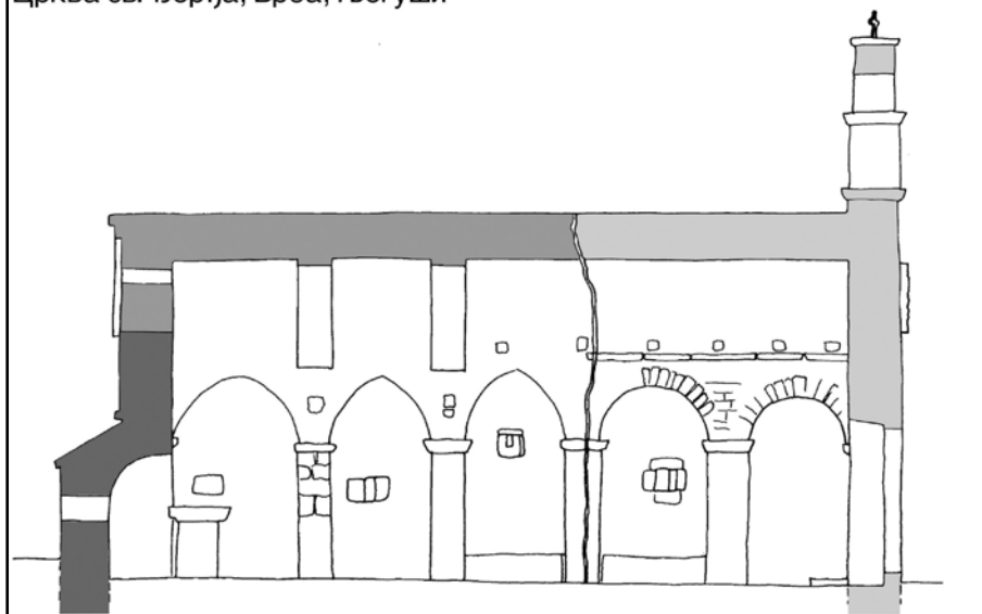
Подужни пресјек са погледом на јужну страну
